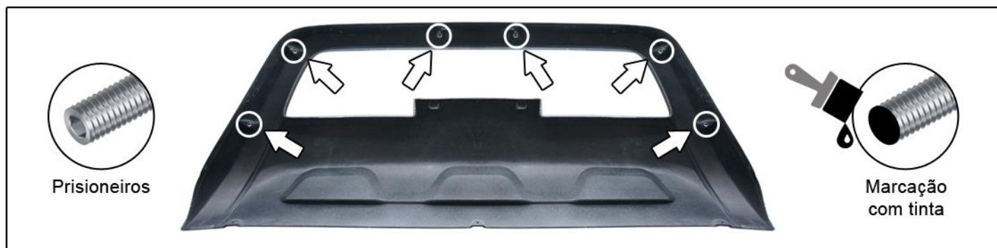
C) Inserir os 6 prisioneiros nos insertos da peça conforme locais indicados. Em seguida, faça uma marcação com tinta na ponta dos prisioneiros (essa marcação serve p/ verificar os locais de furação do para-choque conforme etapa seguinte).
